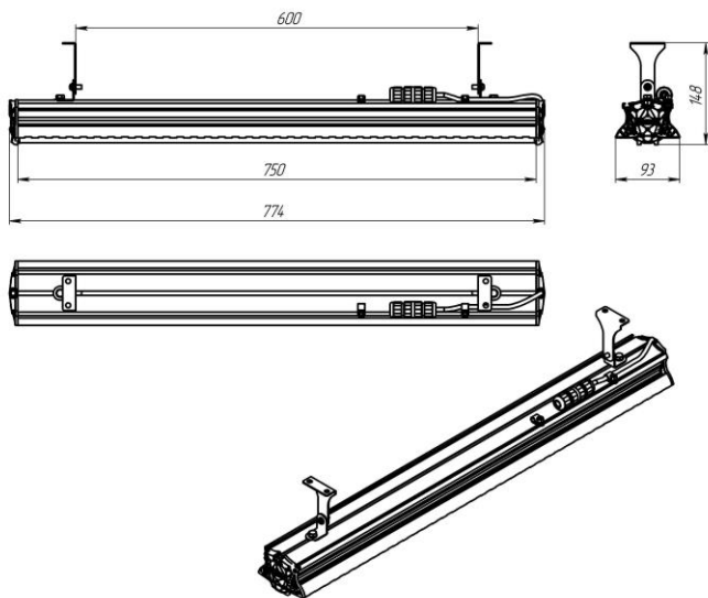
Рисунок 2 Светильник «L-industry 90 Turbine» с поворотным креплением.
